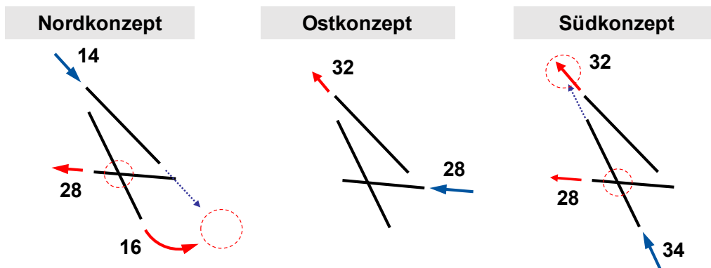
Abbildung 1-1: Flugbetriebskonzepte am Flughafen Zürich
