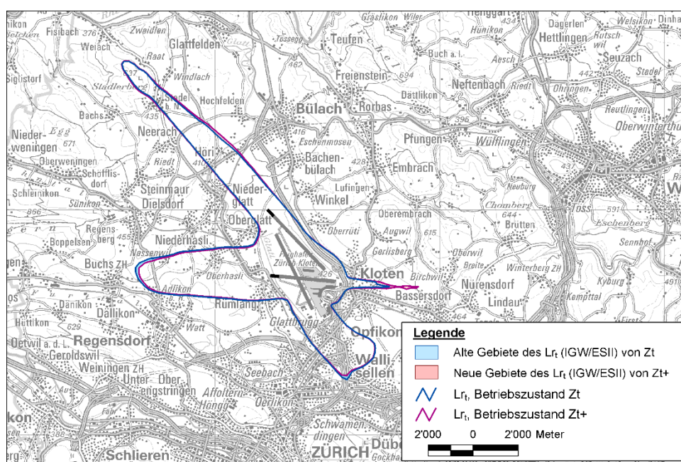
Abbildung 5-1: Beurteilungspegel L_{r1} , dargestellt ist die 60-dB-Kontur (IGW ESII) des Ausgangszustands Zt (blau) im Vergleich zum Betriebszustand Zt+ (magenta). Gebiete des L_{r1} , welche von Zt+ im Vergleich zu Zt entlastet werden, sind blau eingefärbt, und Gebiete des L_{r1} , welche von Zt+ im Vergleich zu Zt zusätzlich belastet werden, sind rot eingefärbt. Karte PK200 reproduziert mit Bewilligung von swisstopo (JA100116).
