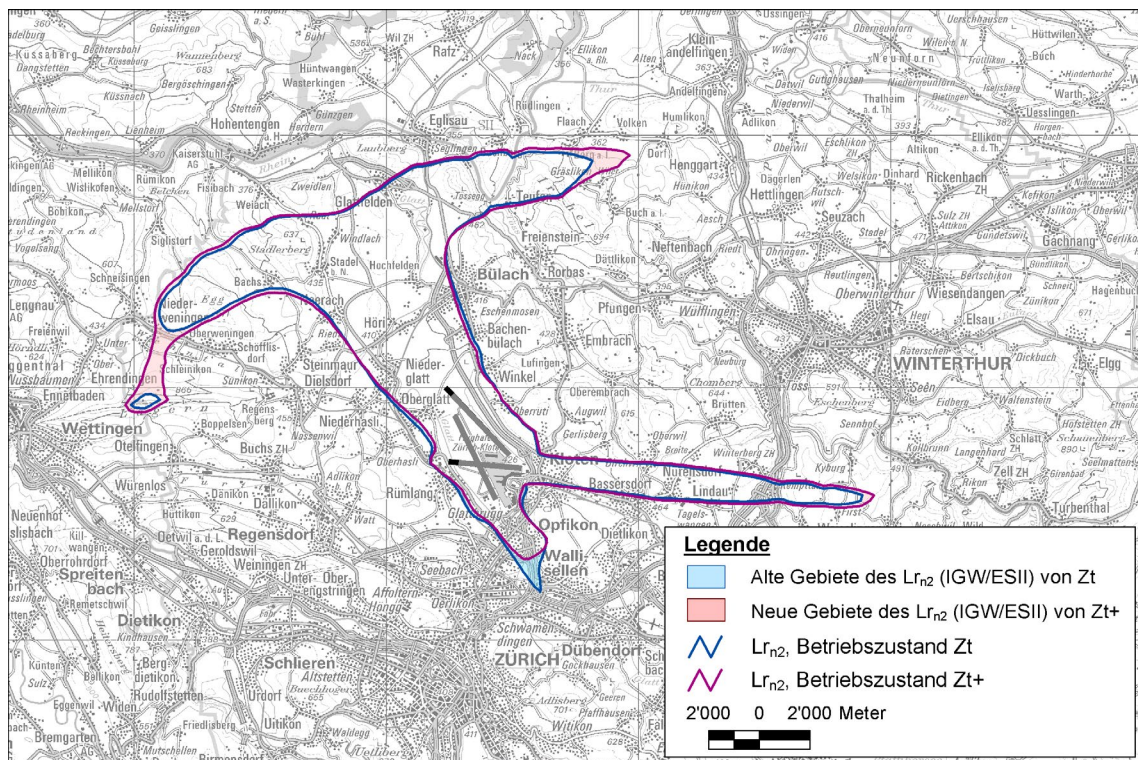
Abbildung 5-3: Beurteilungspegel L_{r,n2} , dargestellt ist die 50-dB-Kontur (IGW ESII) des Ausgangszustands Zt (blau) im Vergleich zum Betriebszustand Zt+ (magenta). Gebiete des L_{r,t} , welche von Zt+ im Vergleich zu Zt entlastet werden, sind blau eingefärbt, und Gebiete des L_{r,t} , welche von Zt+ im Vergleich zu Zt zusätzlich belastet werden, sind rot eingefärbt. Karte PK200 reproduziert mit Bewilligung von swisstopo (JA100116).
