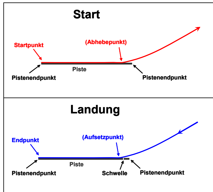
Abbildung 8-2: Definition Start- und Landepunkt der Flugbahnen, welche mit dem jeweiligen Pistenendpunkt (d.h. die Enden der befestigten Piste) zusammenfallen. Der Aufsetzpunkt der Flugbahnen bei der Landung liegt jeweils hinter der Schwelle (in Flugrichtung)
