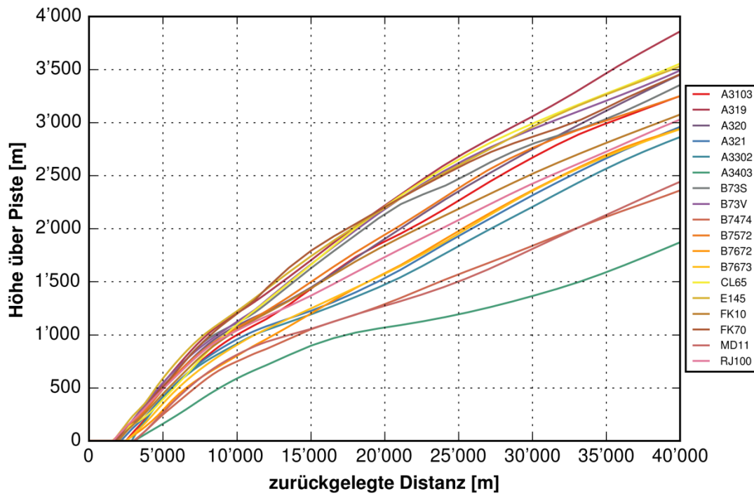
Abbildung 8-19: Höhenprofile Grossflugzeuge, Starts N34
