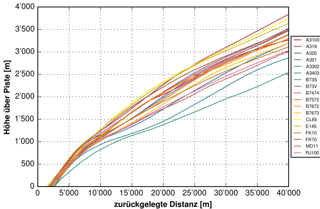
Abbildung 8-15: Höhenprofile Grossflugzeuge, Starts N32
