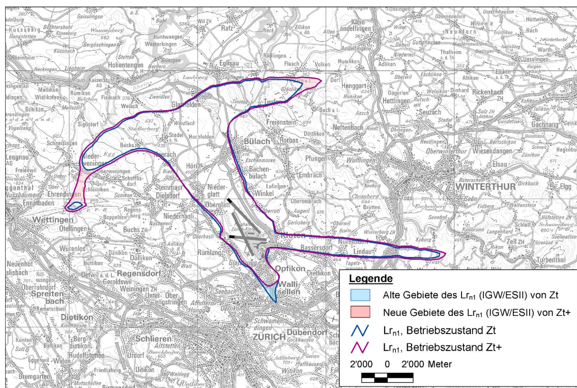
Abbildung 5-2: Beurteilungspegel L_{r_{n1}} , dargestellt als 55-dB-Kontur (IGW ESII) des Ausgangszustands Zt (blau) im Vergleich zum Betriebszustand Zt+ (magenta). Gebiete des L_{r_{n1}} , die von Zt+ im Vergleich zu Zt entlastet werden, sind blau eingefärbt, und Gebiete des L_{r_{n1}} , die von Zt+ im Vergleich zu Zt zusätzlich belastet werden, sind rot eingefärbt. Karte PK200 reproduziert mit Bewilligung von swisstopo (JA100116).
